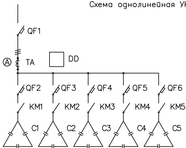
Схема однолинейная УKM 40квар
