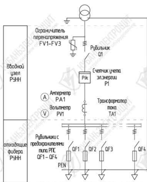
Схема РУНН №01 для КТП с внутренней ячейкой.
